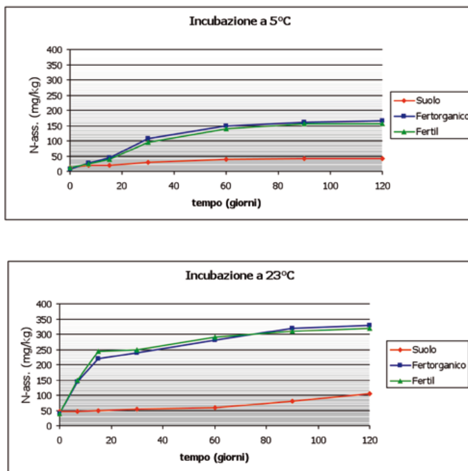
Fig. 5 - Curve di mineralizzazione di FERTIL e FERTORGANICO a 5 e 23° C sviluppate presso il Dipartimento di Scienze e Tecnologie Agroambientali dell' Università di Bologna dal dott. Cavani. Le curve rappresentano il rilascio dell'azoto mineralizzabile nel tempo. Sono curve cumulative apparenti, ovvero tengono conto anche dell'apporto di azoto proveniente dalla mineralizzazione della sostanza organica del suolo.
